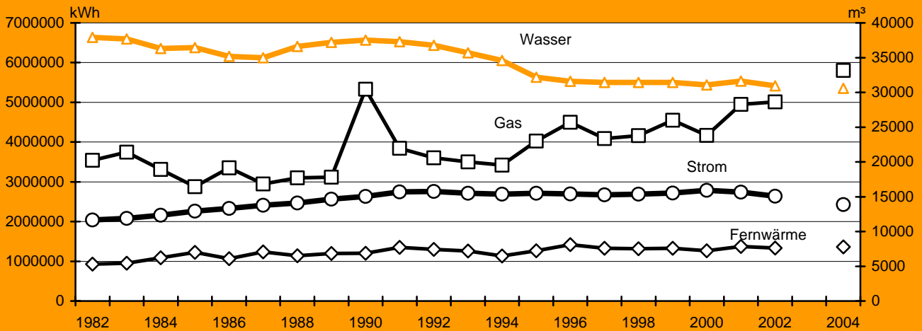
Energie- und Wasserversorgung in 1000 kWh bzw. 1000 m 3
